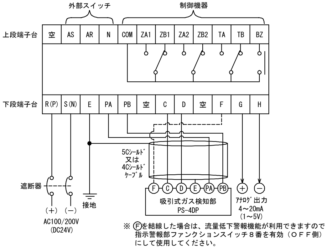
図9 回路図（吸引式検知部 PS-4DP）
