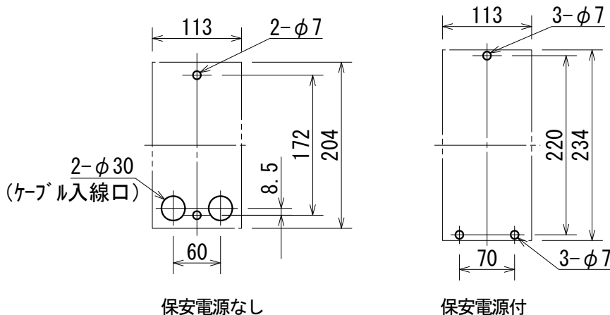
図4 壁掛式 取付穴寸法図
