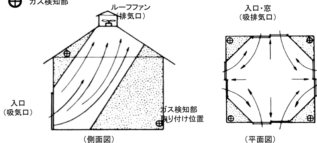
屋内取り付け位置の例
