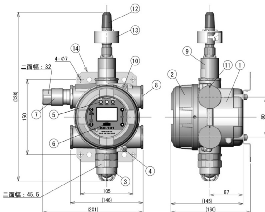
ケーブルグラント取り付け例(左上)
