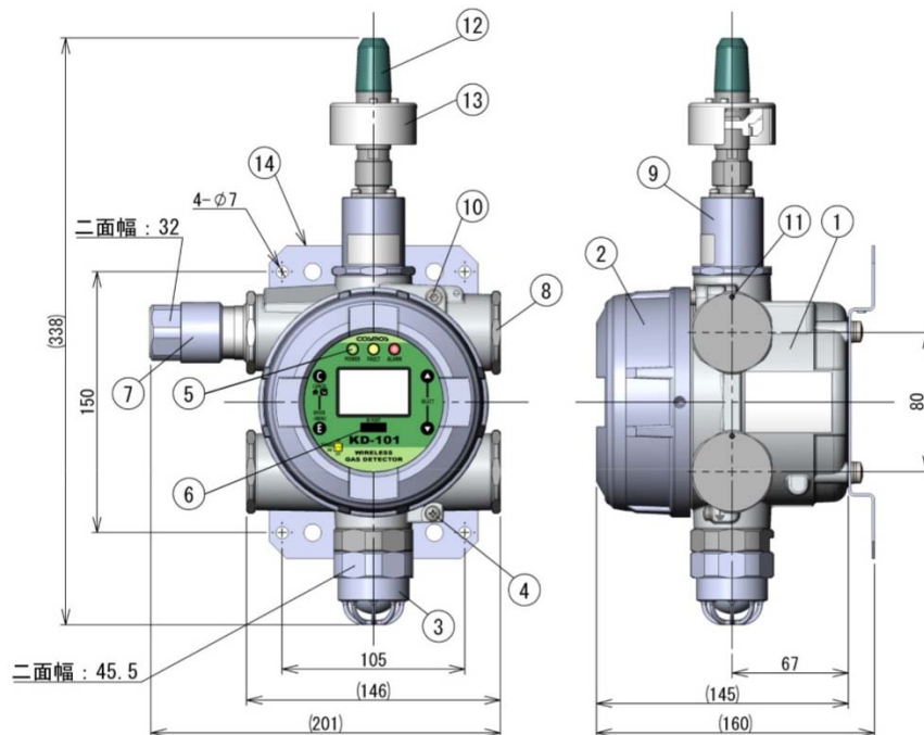
ケーブルグラウンド取り付け例(左上)
