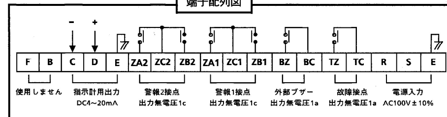
端子配列図
