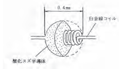
図1. センサ構造
