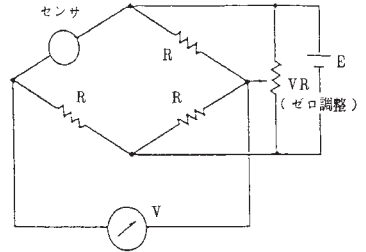
図2. 基本回路
